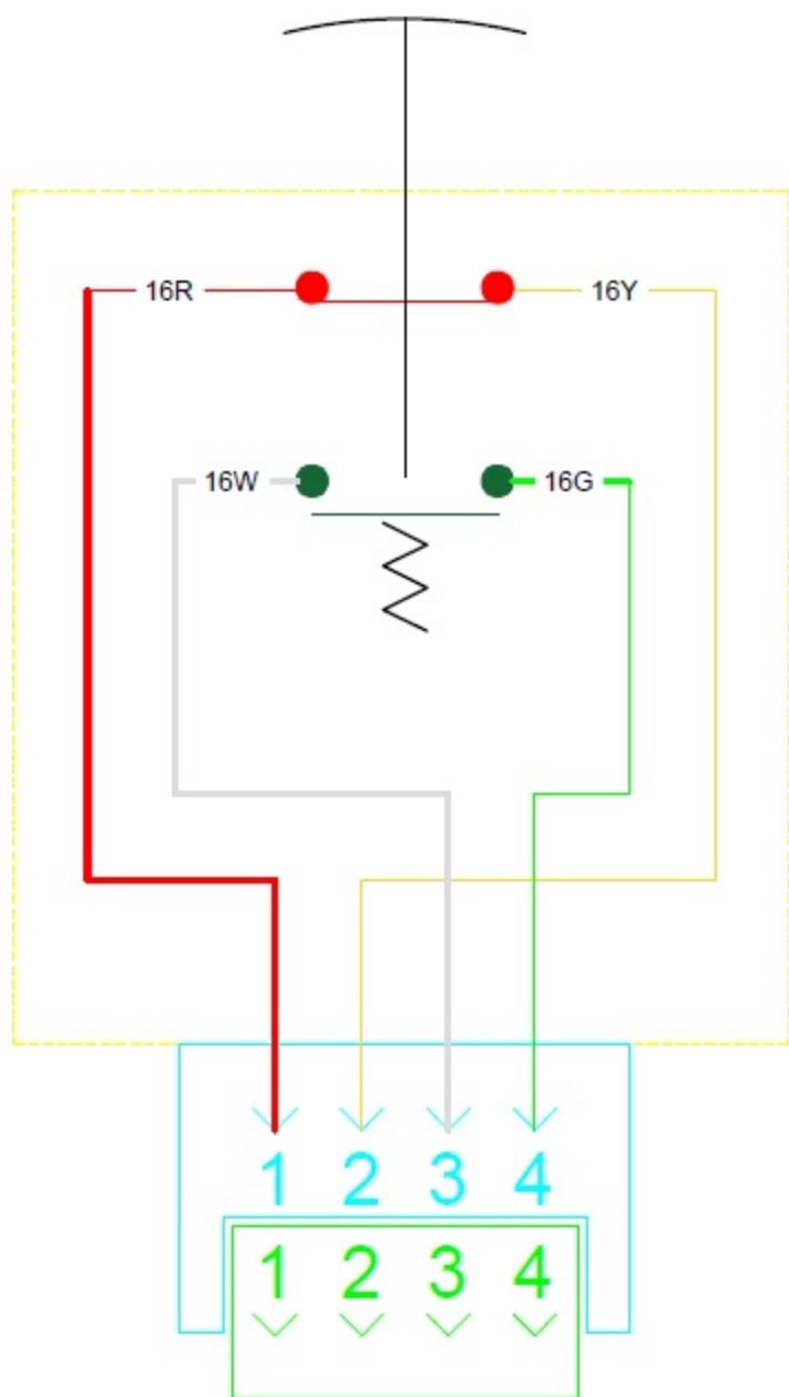
WIRING SCHEMATIC
