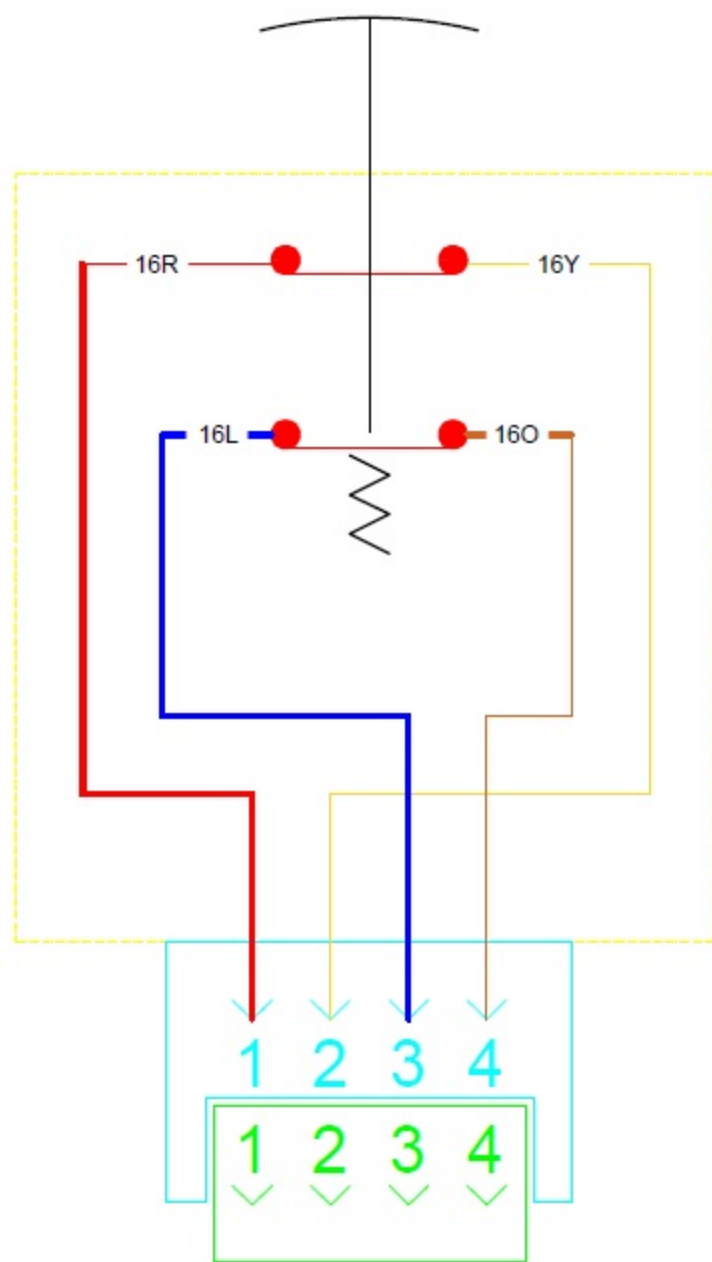
WIRING SCHEMATIC
