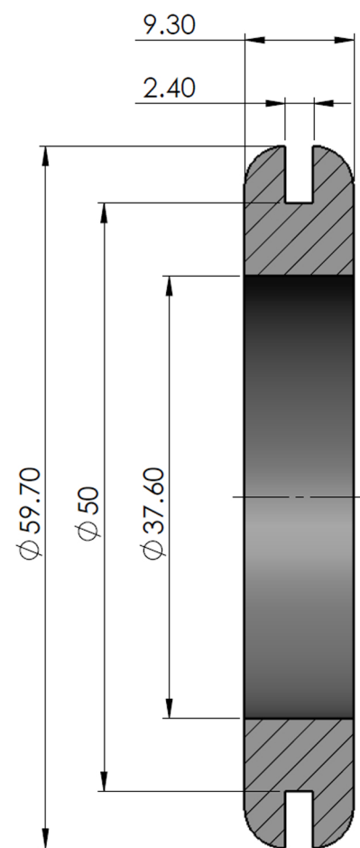
SECTION A-A
