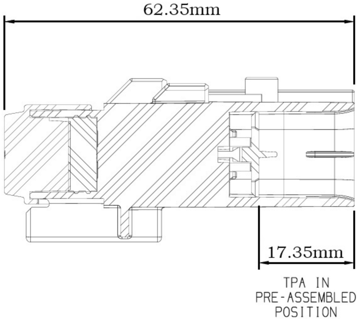
SECTION A-A
