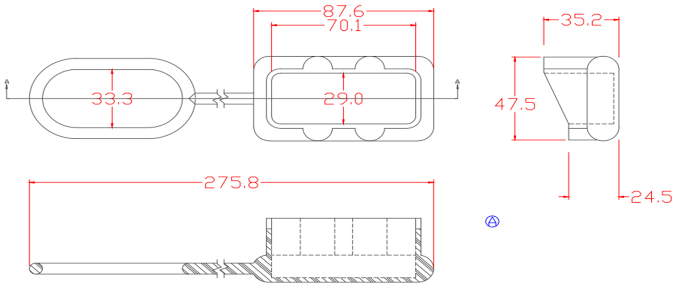
SECTION A-A
