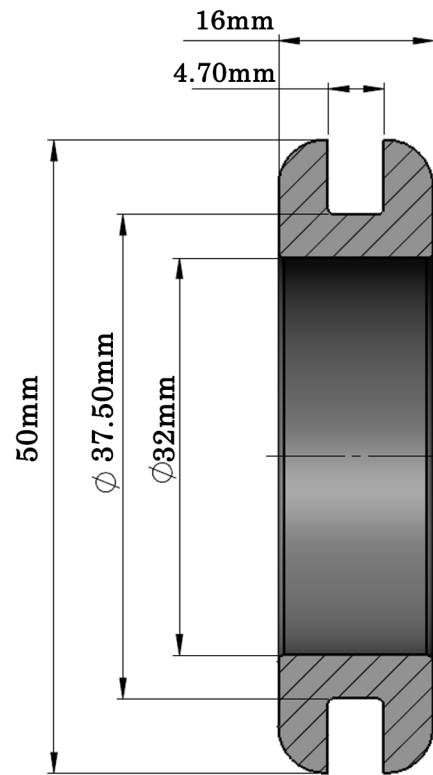
SECTION A-A
